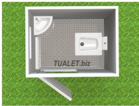
Туалетный модуль T-54
